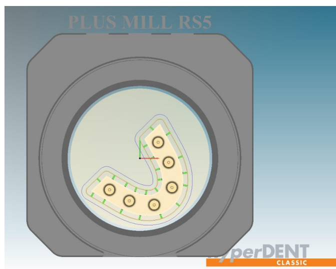
Slika 24. Postavljanje modela u CAM računalnom alatu
