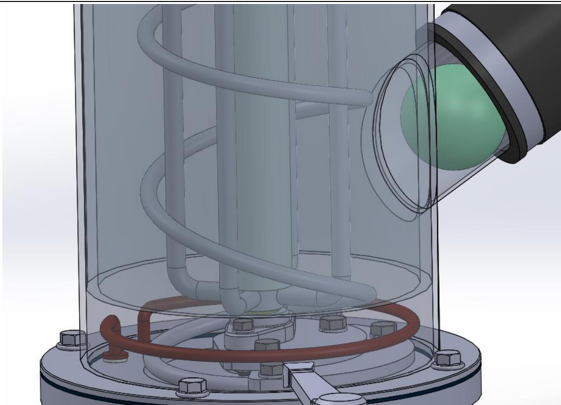
Slika 23. Ulaz golf loptice u prostor za pranje
