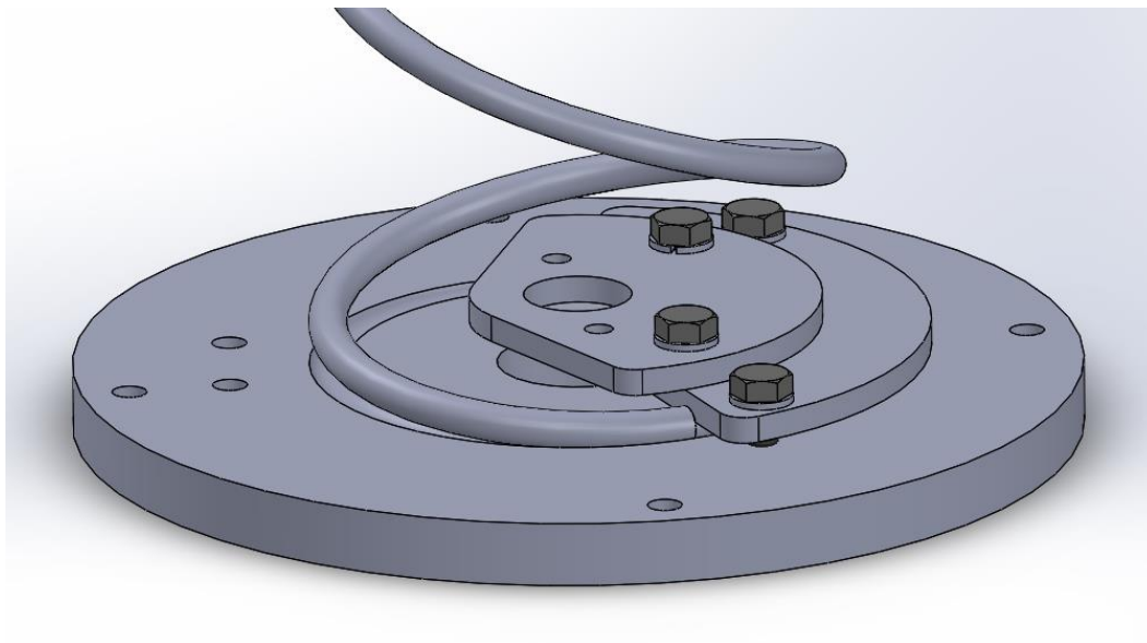
Slika 18. Prihvat spirale za dno
