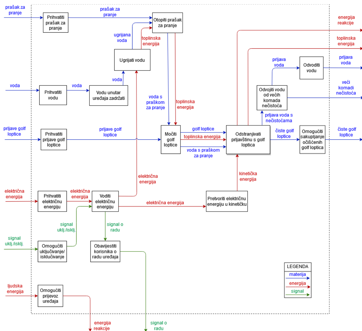
Slika 8. Funkcijska dekompozicija
